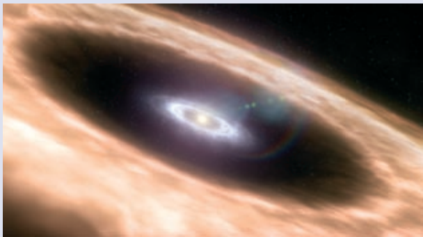
Figuur 2: Schets van een schijf met gas en stof rond een jonge ster. 4 Nieuwe astronomische waarnemingen laten zien dat sommige schijven een gat in hun stofschijf hebben waarin waarschijnlijk al nieuwe Jupiter-achtige planeten zijn gevormd. De afmetingen van de schijf zijn vergelijkbaar met die van ons eigen zonnestelsel. Credit: European Southern Observatory.
