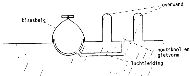
Figuur 19: Bronsoven, doorsnede
