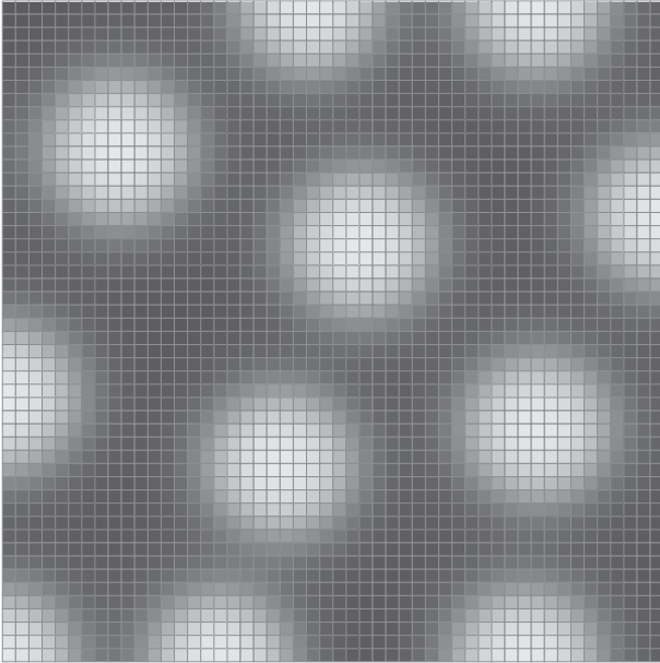
Figuur 2. Een Turing-patroon. Donker: hoge concentratie van morfogen Y; licht: hoge concentratie van X en Y. (simulatie uitgevoerd met ons pakket VirtualLeaf, http://virtualleaf.googlecode.com )
