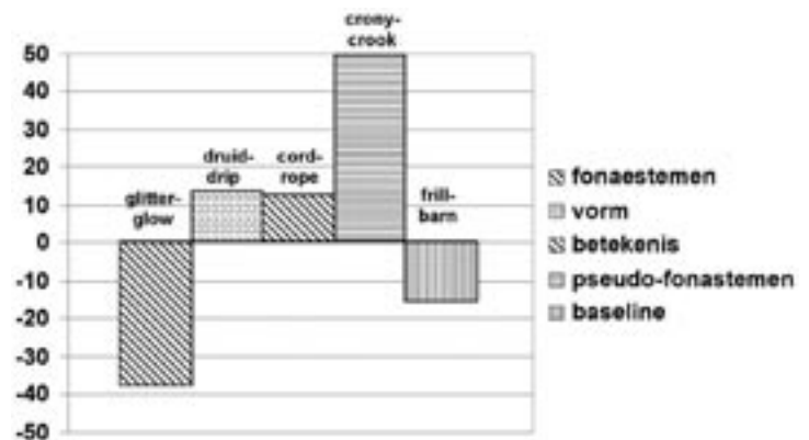
Figuur 1. Primingeffecten (priming-isolatie) in milliseconden (Bergen, 2004)
