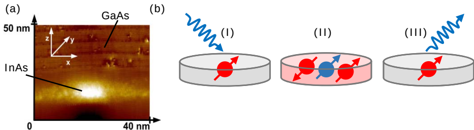
Figuur 9.7: (a) Elektronenmicroscopie afbeelding van een InAs quantum dot (QD) die in een GaAs kristal is ingebouwd. (b) Schematische weergave van de absorptie en emissie van een foton door een QD geladen met een enkel elektron (rode bolletje). Een foton valt (I) op de QD, creëert (II) een elektron en elektrongat (blauw bolletje) paar, en wordt (III) vervolgens weer uitgezonden.
