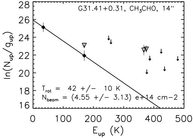
Fig. B.11. RTD fits for \text{CH}_3\text{CHO} .
