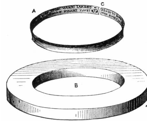
Afb. 4. Schets van de muntring met binnenring om de letters tijdens de muntslag op de rand van de rondel of het muntplaatje te zetten. Bron: Ansell, A Treatise on Coining 25, figuur 19.
