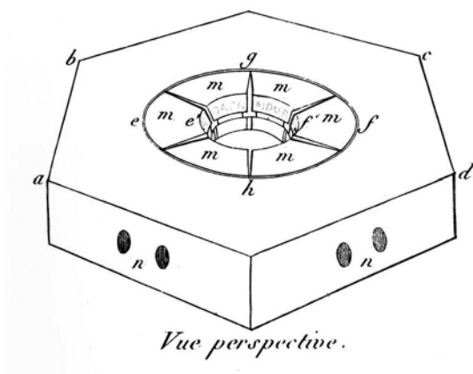
Afb. 5 Een deelbare muntring volgens een ontwerp van J. Droz. Bron: J.M. Darnis Le graveur-mecanicien Jan Pierre Droz 1er adapteur des viroles pleines et brisées aux mecanismes du balancier monétaire (1982).
