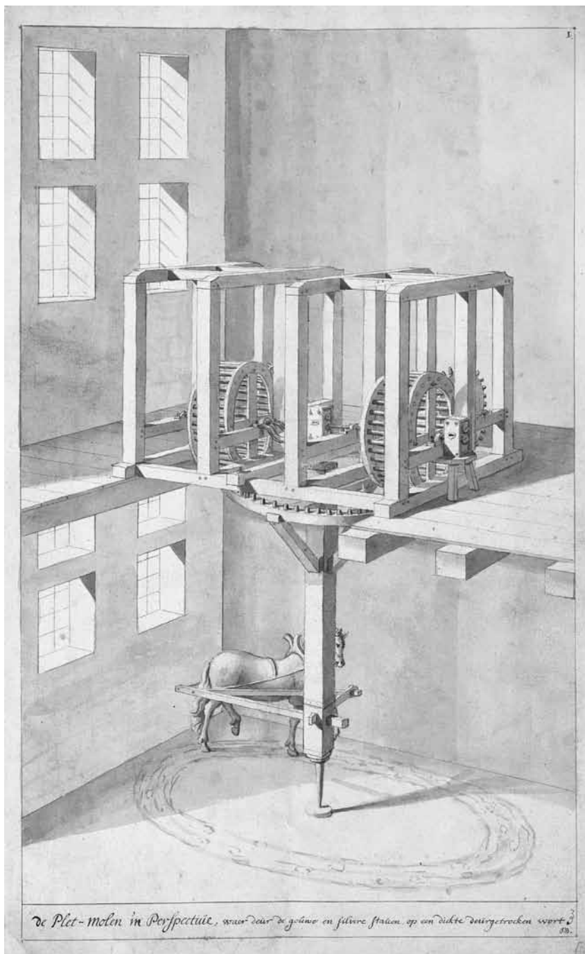
Afb. 11. Tekening van een paardentred voor de Zeeuwse Munt door Daniël de Blicq, 1671. Zeelandia Illustrata , ZI III 1027-02.
