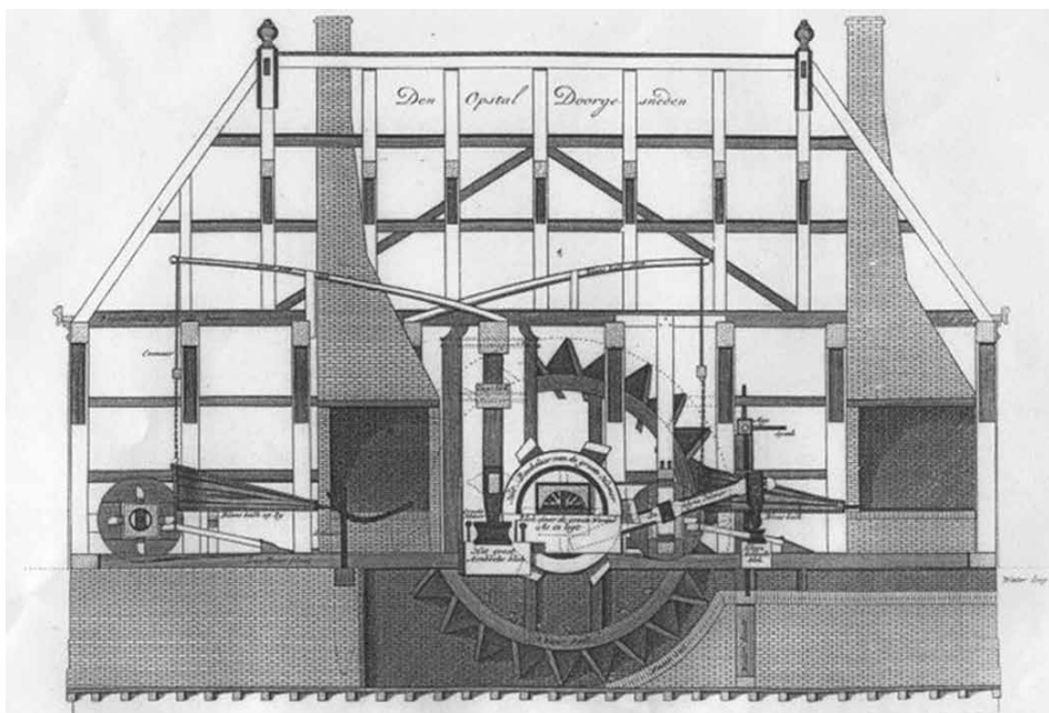
Afb. 30. Doorsnede van een door waterkracht aangedreven kopermolen. Zichtbaar is het door het water aangedreven rad dat de blaasbalgen voor de twee ovens in beweging brengt.
