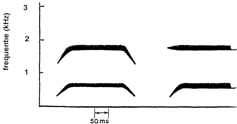
Figuur 10 Gestileerd verloop van F_1 en F_2 , geschikt als recept voor herkenbare synthese van de syllabereeks [bebde]. In een medeklinkeropenvolgving als [-bd-] is de F_1 -aanduiding van de eerste syllabe bepalend voor de waargenomen articulatieplaats van de [-b] en de F_2 -beginbuiging van de tweede syllabe bepalend voor de [d].
