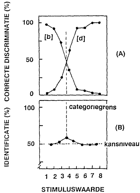
Figuur 14 A categorisatie en B discriminatie langs een [ba] - [da] continuum. Categoriale waarneming is duidelijk alleen als de syllaben in een vergelijkingspaar uit verschillende tonetische categorieën komen, worden ze (boven kans) gediscrimineerd (naar Studdert-Kennedy, 1976)
