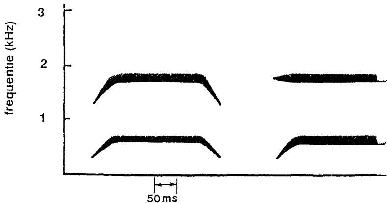
Figuur 10 Gestileerd verloop van F 1 en F 2 , geschikt als recept voor herkenbare synthese van de syllabereeks [bebde]. In een medeklinkeropenvolgving als [-bd-] is de F 1 -aanbuiging van de eerste syllabe bepalend voor de waargenomen articulatieplaats van de [-b] en de F 2 -beginbuiging van de tweede syllabe bepalend voor de [d].
