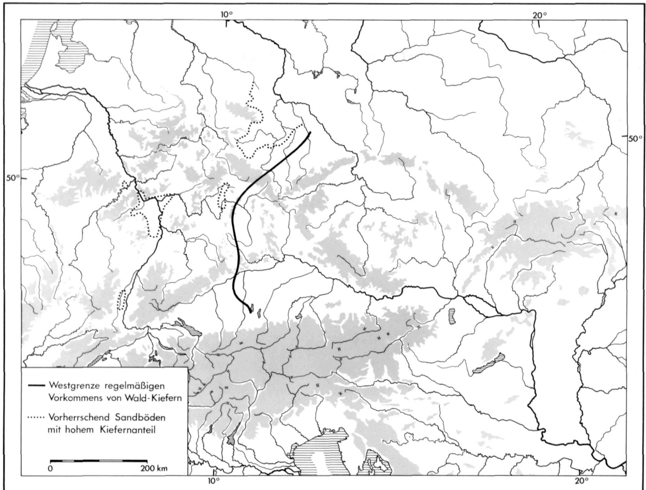
Fig. 77 Westgrenze regelmäßiger Beimengung von Wald-Kiefern (nach: Firbas 1949) während der älteren Nachwärmezeit, also in der ersten Hälfte des Subatlantikums (Firbas Pollenzone IX).
